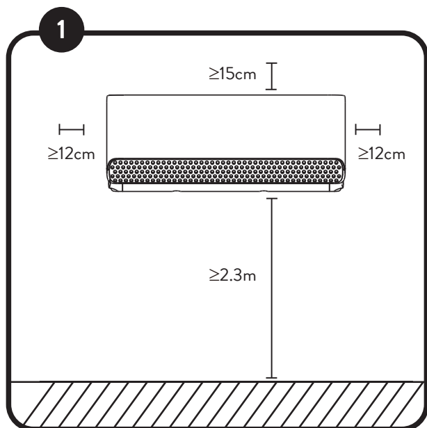
Seleccione el lugar de la instalación
