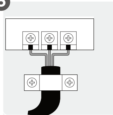
Conecte el cableado (Esto puede no ser necesario en algunos lugares de Norteamérica)
