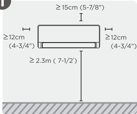
Selección del lugar de instalación
