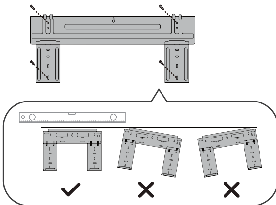
Orientasi Plat Pemasangan yang betul
